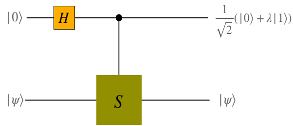
شکل ۱۵: یک مدار ساده که تشخیص می دهد آیا حالت |\psi\rangle برای پایدارساز S که یک عملگر یکانی است ویژه مقدارش یک است یا منهای یک.
