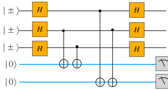
شکل ۳: یک مدار ساده که مداری که خطای فاز-برگردان را تشخیص می دهد.
