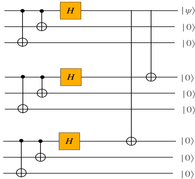
شکل ۷: مداری که حالت کد شده شُر را به حالت اولیه بازمی گرداند، دقیقاً وارون علمگری است که کد شُر را ایجاد می کند.
