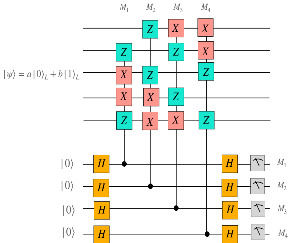
با توجه به این مدار و این شیوه تشخیص ویژه مقدارهای پایدارسازها براحتی معلوم می شود که مدار تشخیص خطا برای کد پنج کیوبیتی مطابق شکل (۱۶) است.
