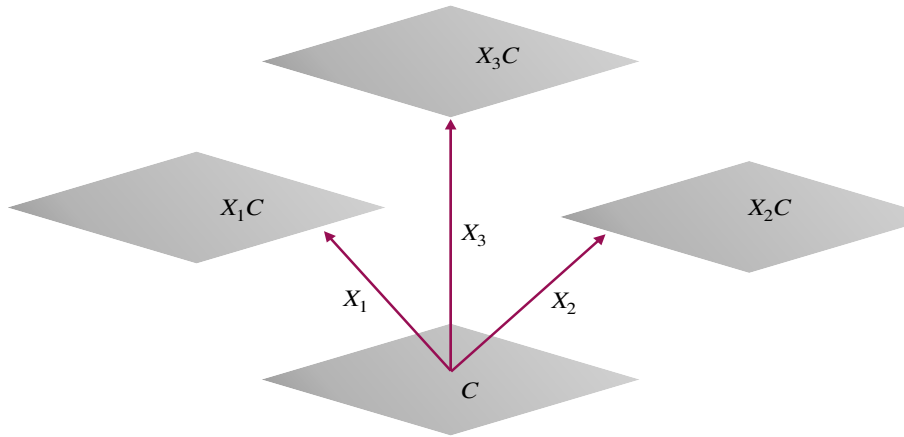
شکل ۱: زیر فضای کد و زیر فضاهایی که در اثر خطا بوجود می آیند.
