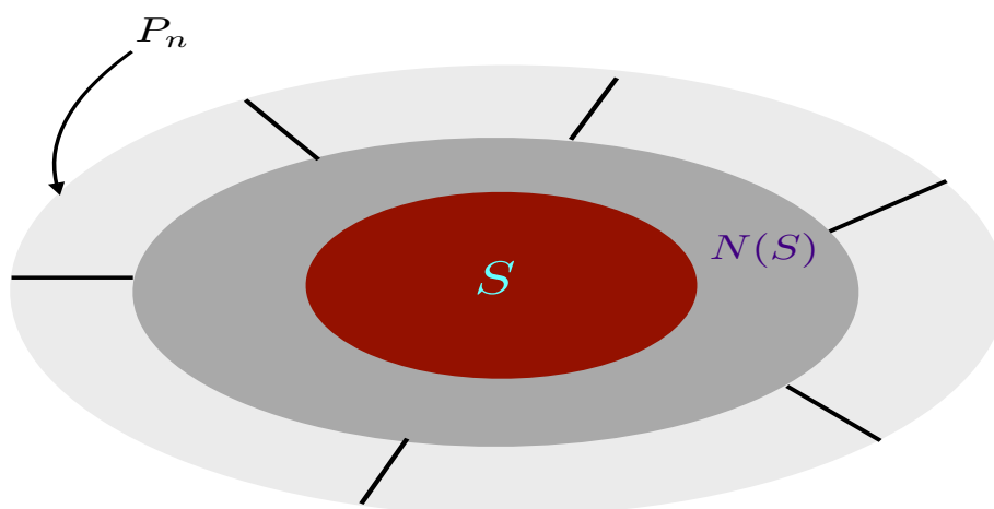
شکل ۱۰: گروه پاوولی، زیرگروه پایدارساز و گروه بهنجارساز این زیرگروه
