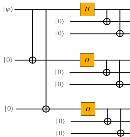
شکل ۵: مداری که کد شر را می سازد.
