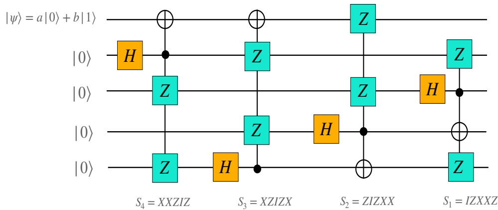
شکل ۱۴: یک مدار کوانتومی که با استفاده از رابطه (۷۹) مداری که کد پنج کیوبیتی را می سازد.
