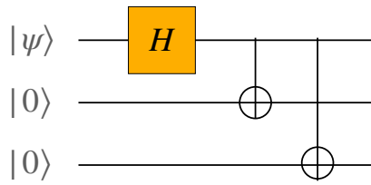
شکل ۴: یک مدار ساده که تبدیل (۳۳) را انجام می دهد.
