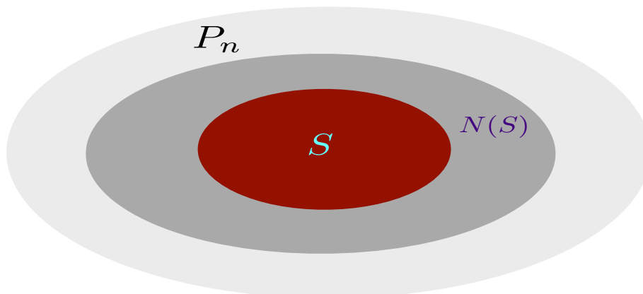
شکل ۸: گروه پاولی، زیرگروه پایدارساز و گروه بهنجارساز این زیرگروه
