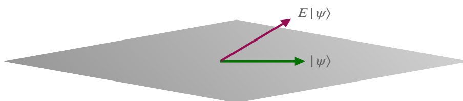
شکل ۱۱: خطاهای قابل شناسایی آنها می هستند که حالت را از فضای کد خارج می کنند و از خود نشانه باقی می گذارند.
