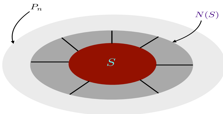
شکل ۹: گروه پائولی، زیرگروه پایدارساز و گروه بهنجارساز این زیرگروه
